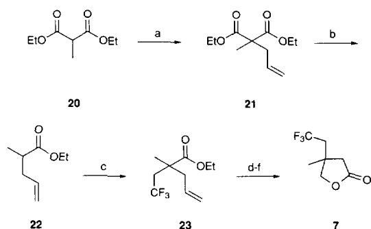
Scheme 2. (a) NaH, \text{CH}_2=\text{CHCH}_2\text{Br} , THF; (b) DMSO/ \text{H}_2\text{O}/\text{NaCl} , \Delta ; (c) LDA, \text{CF}_3\text{CH}_2\text{I} , THF; (d) \text{O}_3 1:1 MeOH/ \text{CH}_2\text{Cl}_2 , -78^{\circ}\text{C} ; (e) Jones oxidation; (f) DIBALH, toluene, -78^{\circ}\text{C} .
