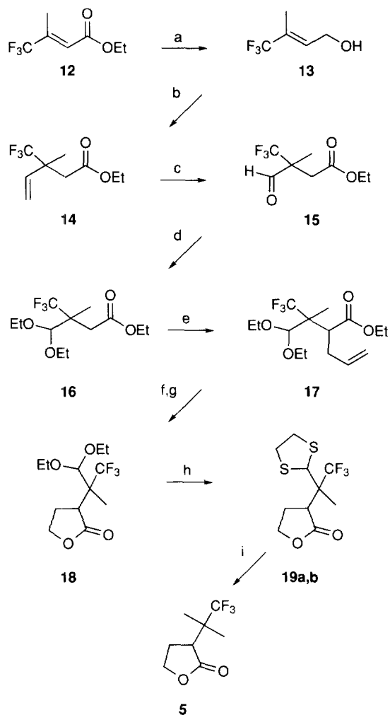
Scheme 1. (a) DIBALH, hexanes, -25^{\circ}\text{C} ; (b) \text{CH}_3\text{C}(\text{OEt})_3 , \text{CH}_3\text{CH}_2\text{COOH} , \Delta ; (c) \text{O}_3 , \text{CH}_2\text{Cl}_2 , -78^{\circ}\text{C} ; (d) \text{HC}(\text{OEt})_3 , p\text{-TsOH} ; (e) LDA, \text{CH}_2=\text{CHCH}_2\text{Br} , THF; (f) \text{O}_3 , \text{CH}_2\text{Cl}_2 , -78^{\circ}\text{C} ; (g) \text{NaBH}_4 , EtOH; (h) \text{HSCH}_2\text{CH}_2\text{SH} , \text{BF}_3 \cdot \text{HOAc} ; (i) Raney Ni, EtOH, \Delta .
